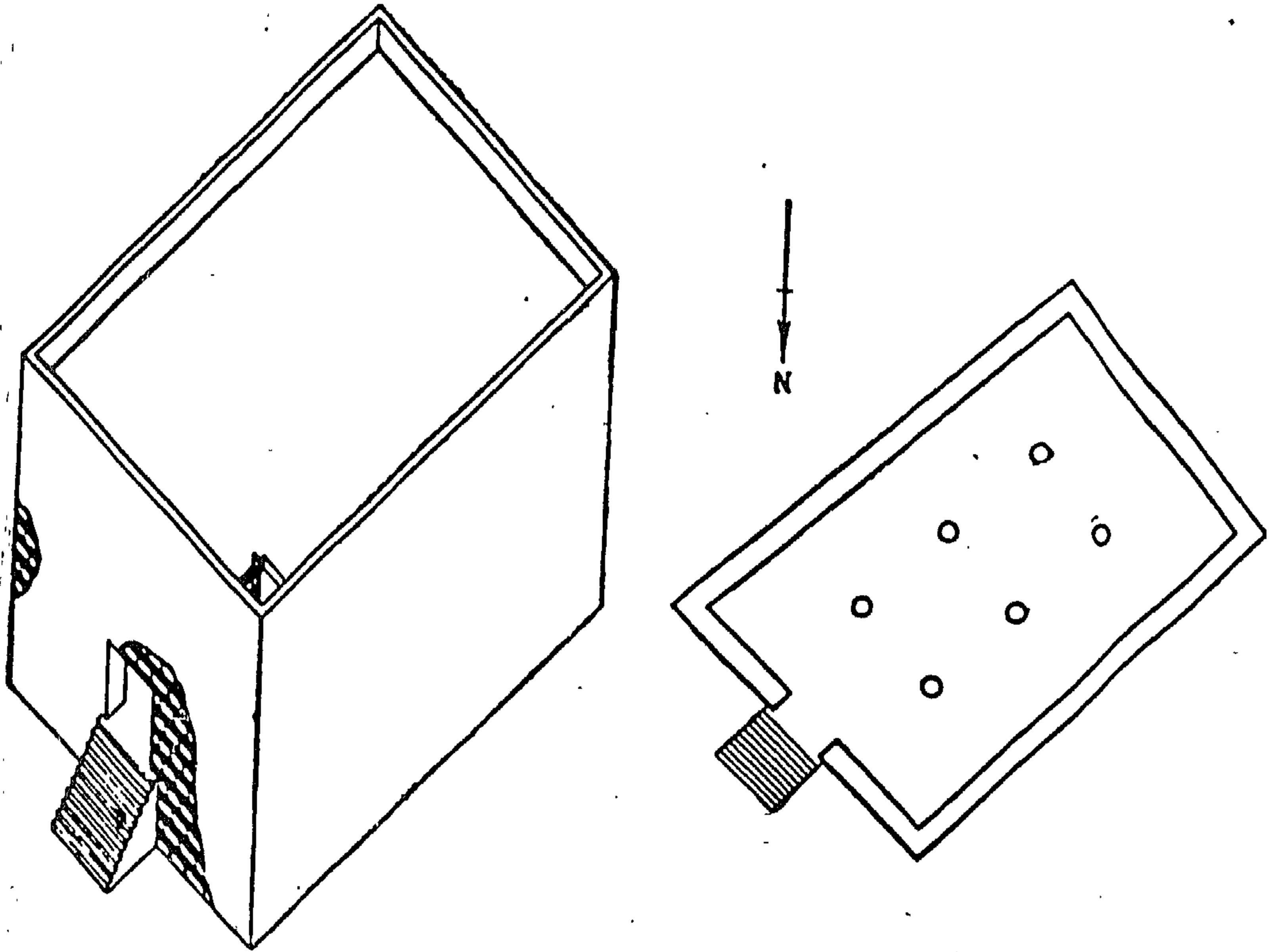
مخطط (١) - مكة المكرمة منظور ومسقط الكعبة في شباب الرسول
